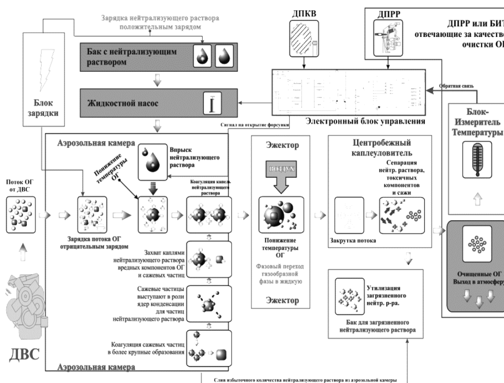
Рисунок 2. – Принцип работы УООГ.
