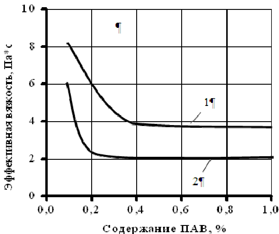
Рисунок 2 – Влияние дозировки ПАВ на вязкость шоколадной массы при градиенте скорости 30 с -1 : 1 - ПАФ; 2- БАД «Витол»
