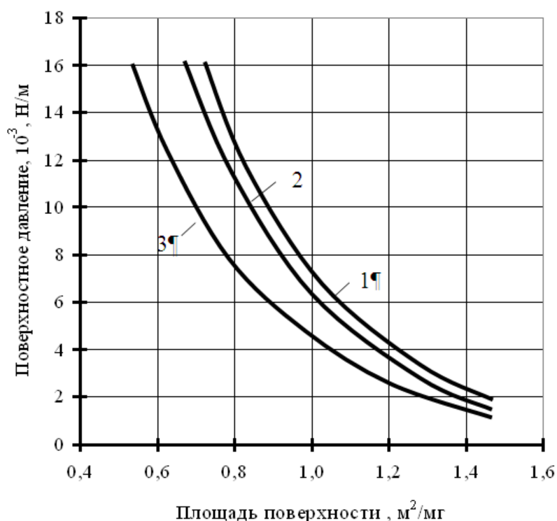
Рисунок 3 – Изотермы поверхностного давления пленок различных ПАВ на воде: 1 - БАД «Витол», 2- ПАФ; 3- СФК (контроль)
