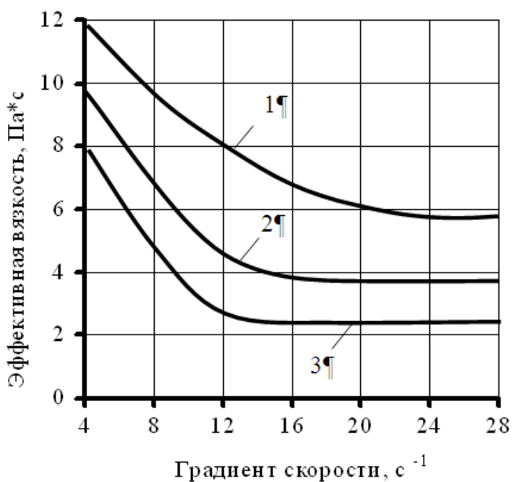
Рисунок 1 – Зависимость изменения эффективной вязкости шоколадной массы от градиента скорости при введении 0,4 % ПАВ: 1 – СФК (контроль); 2- ПАФ; 3- БАД «Витол»
